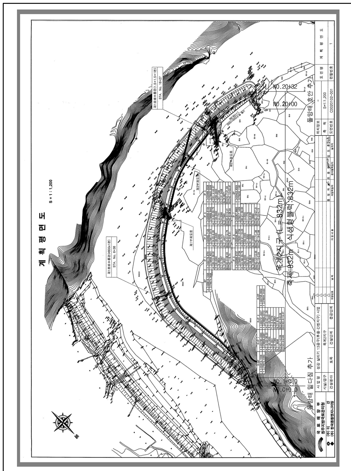
【그림 II.2-2】 옥계2제 계획 평면도
